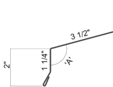
Eave Drip Edge 2" Face
